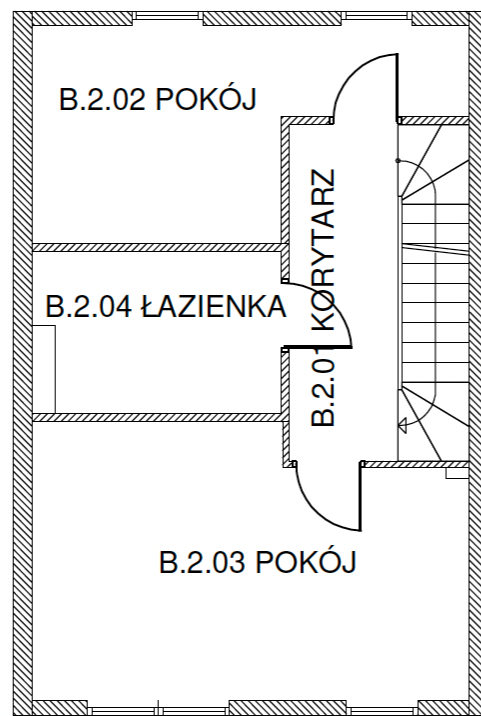
PIĘTRO 1 - 40.91 [m2]
