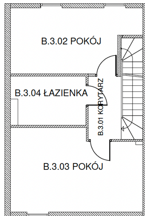
PIĘTRO 2 - 35.90 [m2]
