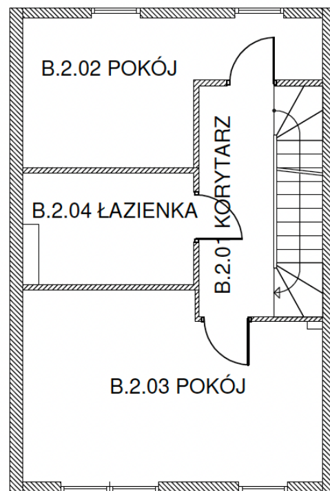
PIĘTRO 1 - 40.91 [m2]
